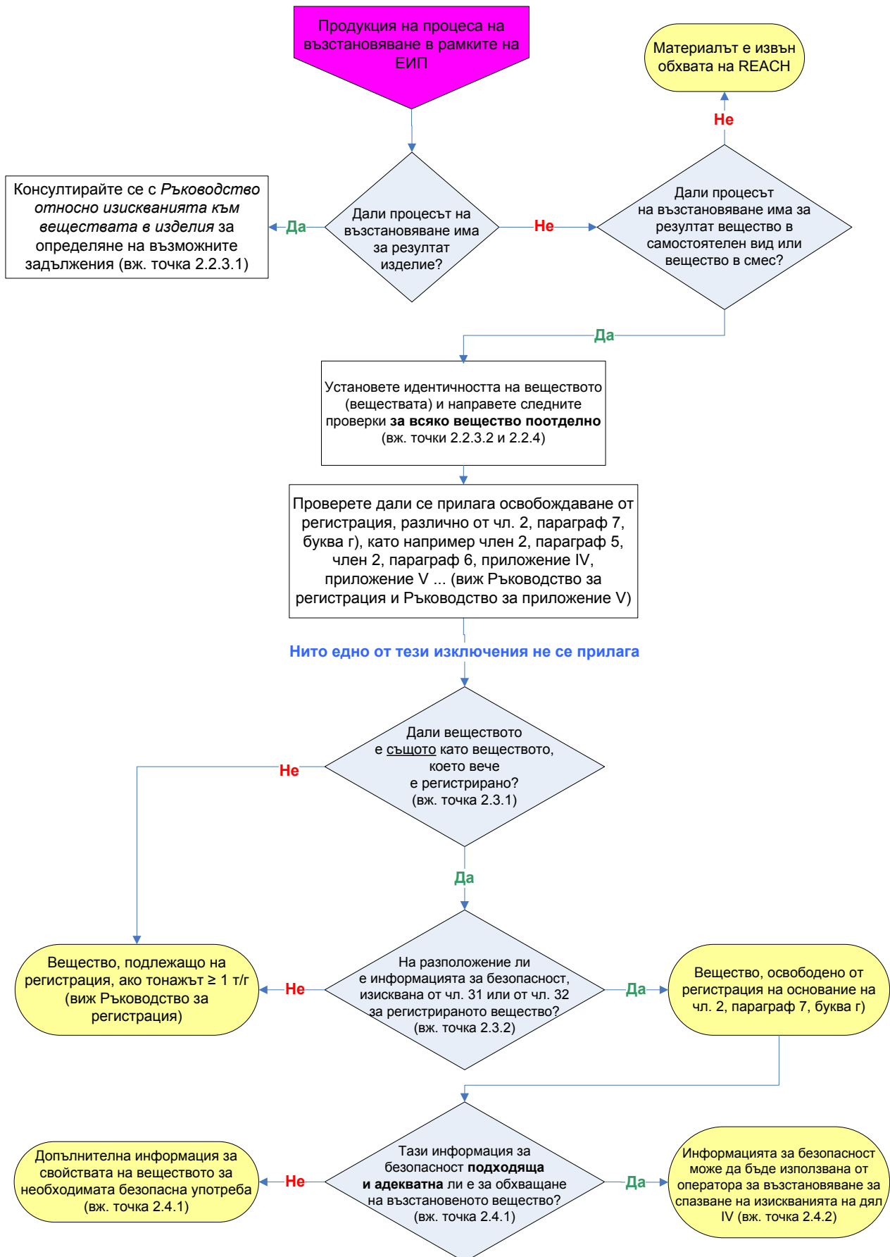
Фигура 2: Работен процес за проверка дали даден оператор по възстановяването може да се позове на член 2, параграф 7, буква г) от REACH и свързаните с това задължения
